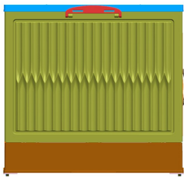
左视图
